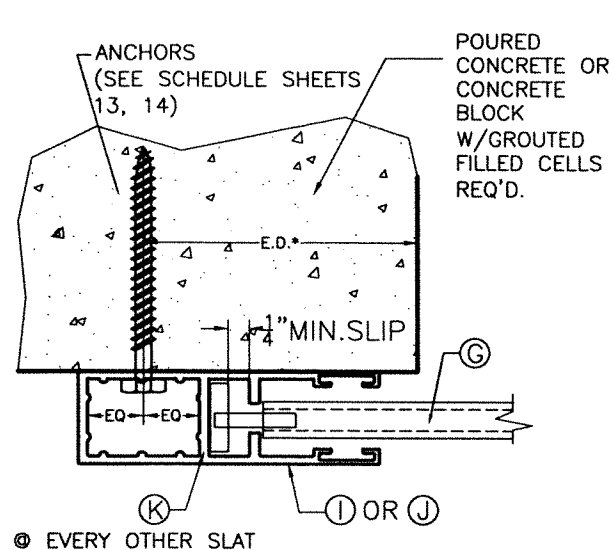
SECTION J-J : WALL MOUNT
