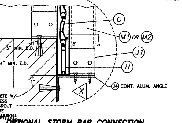
OPTIONAL STORM BAR CONNECTION SCALE : N.T.S
