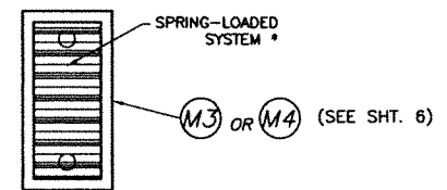
SECTION S - S : SINGLE STORM BAR SCALE : N.T.S
